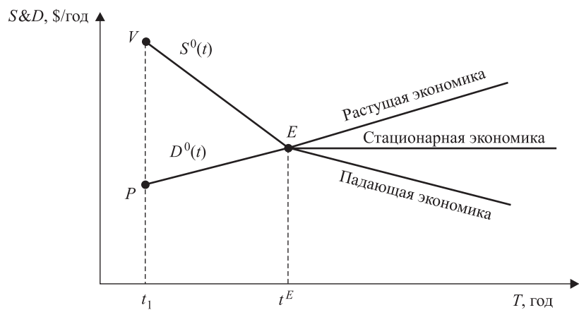
Рис. 6. Классические стационарная и нестационарные двухагентные рыночные экономики в координатной системе [T, S\&D]
