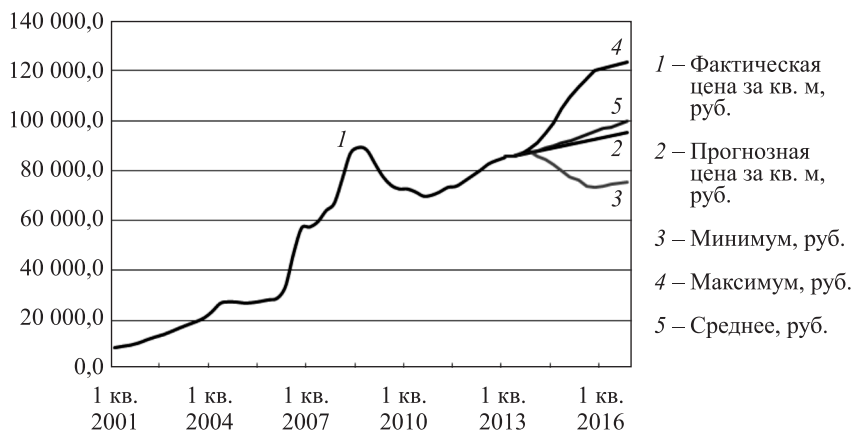
Рис. 3. Сравнение результатов имитационного моделирования Монте-Карло и первичной экстраполяции цен за кв. метр (методом Хольта)
