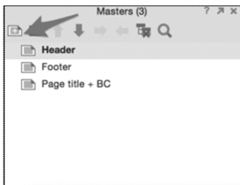
Рис. 2. Панель «Masters»
