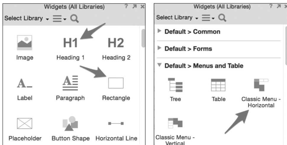
Рис. 3. Панель «Widgets»
